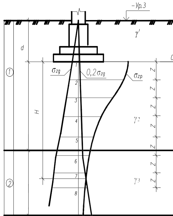
Схема к расчету осадки по методу линейно деформируемого полупространства
