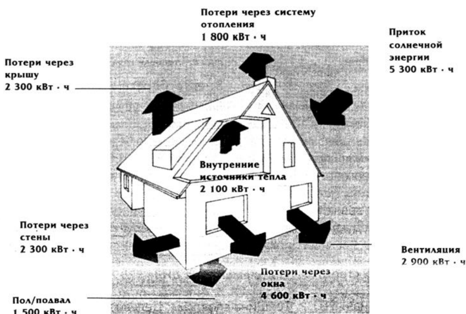
Рис.8.2. Годовые приток и потери энергии дома (всоответствие с ДНЭ критериями).
