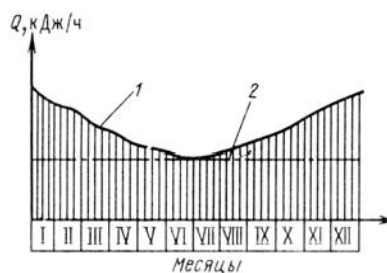
Рис.2.3. Годовой график потребления теплоты потребителем: 1- неравномерное; 2 - равномерное
