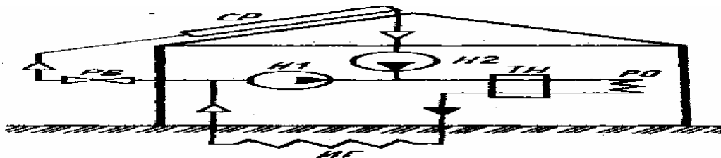
Рис.4.3 Схема с комбинированным использованием теплоты грунта и солнечной радиации
