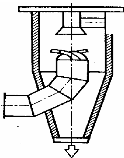
Рис. 7.5. Прямоточный циклон ЦКТИ.
