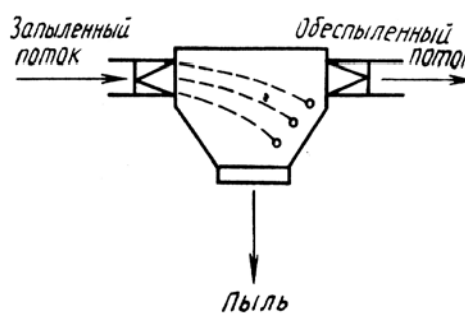
Рис.7.4. Пылеосадительная камера
