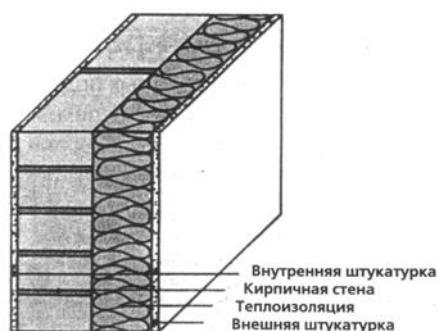
Рис.8.3 Утепленная стена («Термошуба»)
