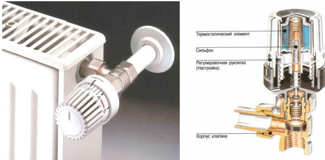
Рис.8.8 Радиаторный термостат
