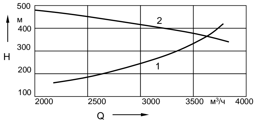
1 – характеристика трубопровода; 2 – характеристика насосной станции
