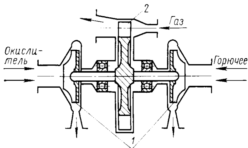
Рисунок 1 – Схема турбокомпрессорного агрегата
